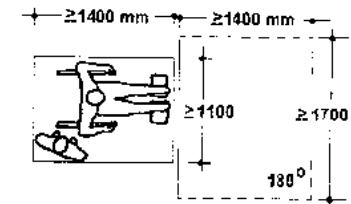
LIFTKABIN ÉS LIFTELŐTÉR AKADÁLYMENTES HELYSZÜKSÉGLETE
