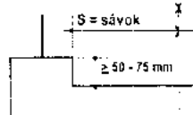
AKADÁLYMENTES LEJTŐ, RÁMPA PEREM ÉS LÉPCSŐFOK METSZET
