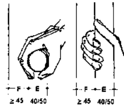
VÍZSZINTES- ÉS FÜGGŐLEGES KORLÁT ELHELYEZÉS (mm)
