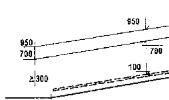
LEJTŐK-, RÁMPÁK-, ÉS LÉPCSŐKORLÁTOK MAGASSÁGA (mm)
