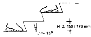
AKADÁLYMENTES LEJTŐ, RÁMPA PEREM ÉS LÉPCSŐFOK METSZET
