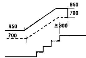
LEJTŐK-, RÁMPÁK-, ÉS LÉPCSŐKORLÁTOK MAGASSÁGA (mm)
